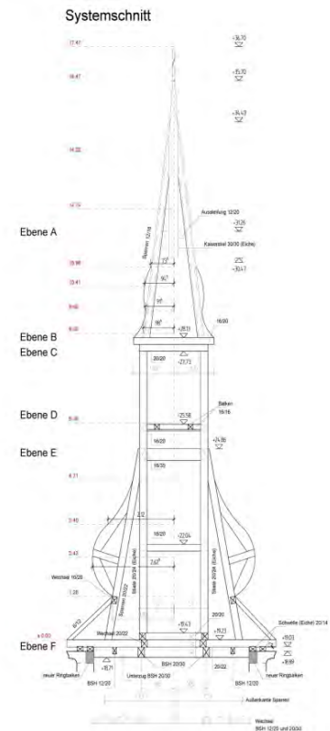
Schnitt / Visualisierung / neue Turmhaube
