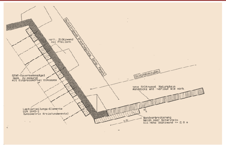
Grundriss zur Sanierung der Stützwände
